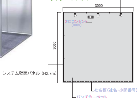
1小間 平面図
