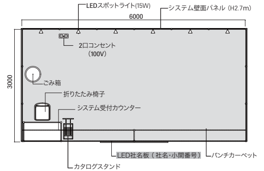
2小間 平面図
