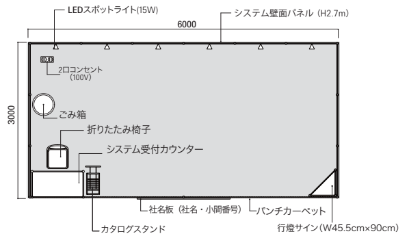
2小間 平面図
