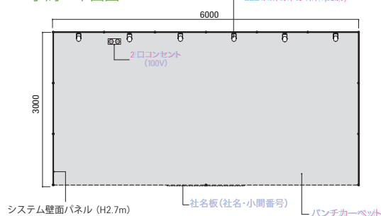
2小間 平面図
