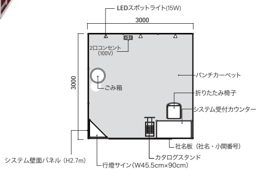
1小間 平面図
