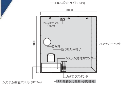
1小間 平面図
